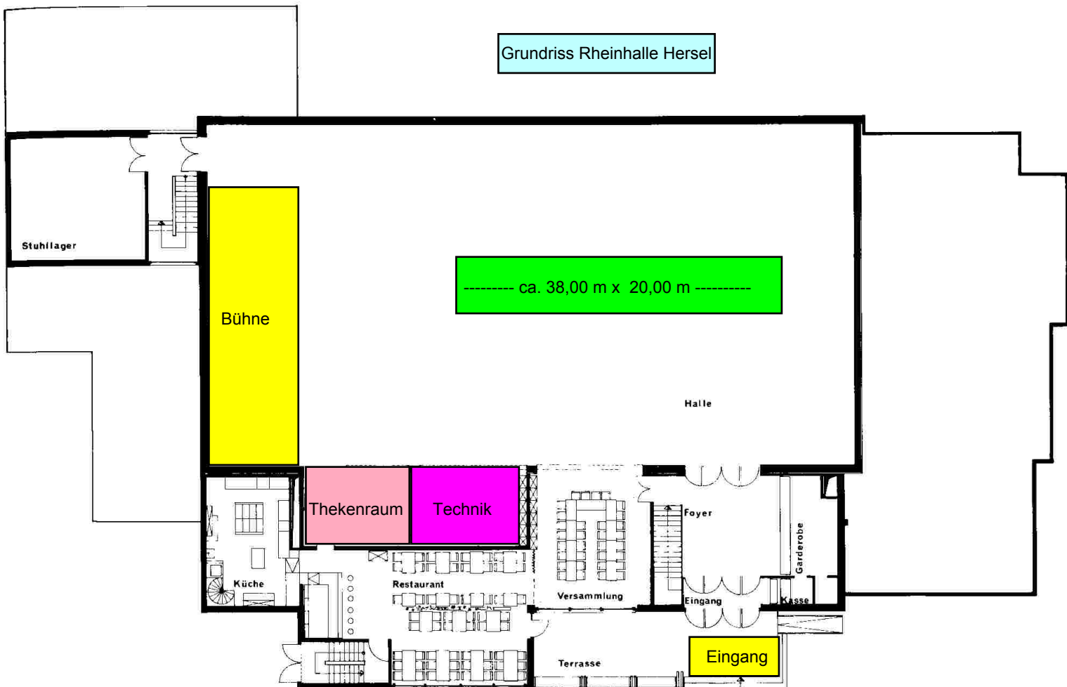
Grundriss Erdgeschoss
